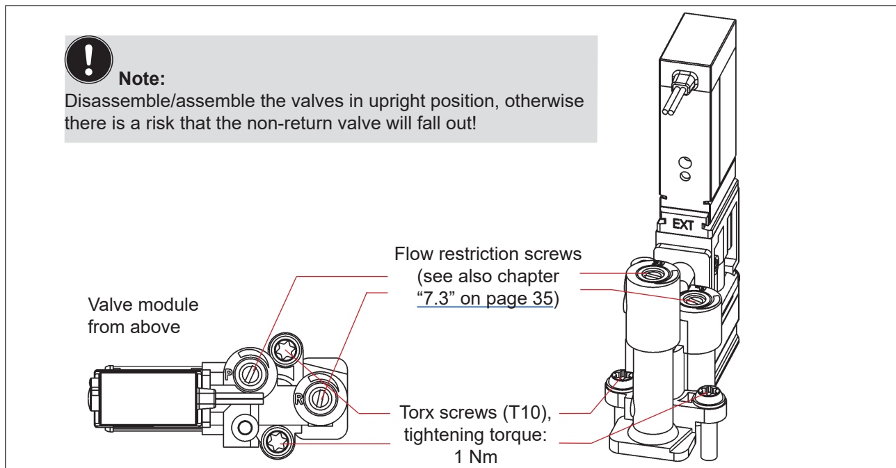
Fig. 38: Valve module Type 6524
